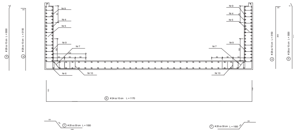
Zbrojenie ściany i płyty dennej odcinka 2
