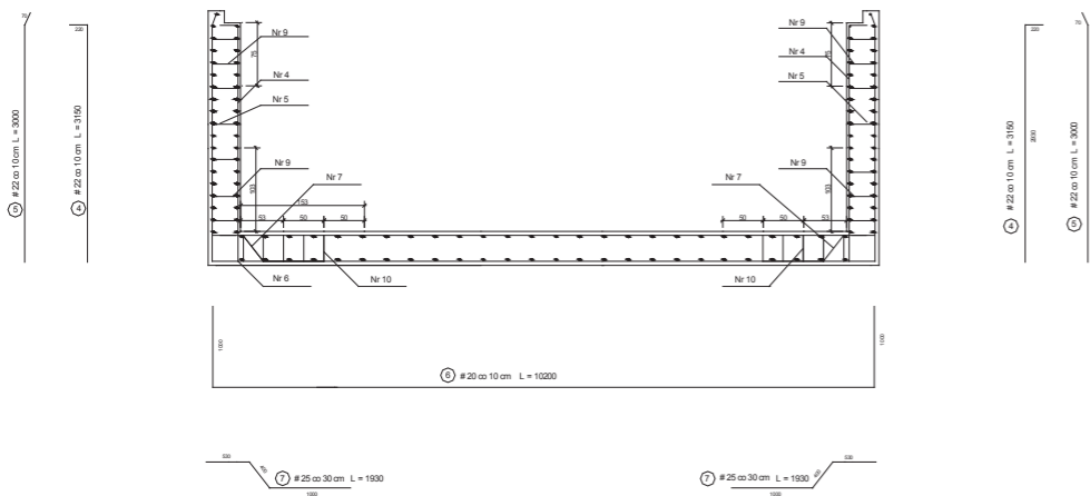
Zbrojenie ściany i płyty dennej odcinek 1
